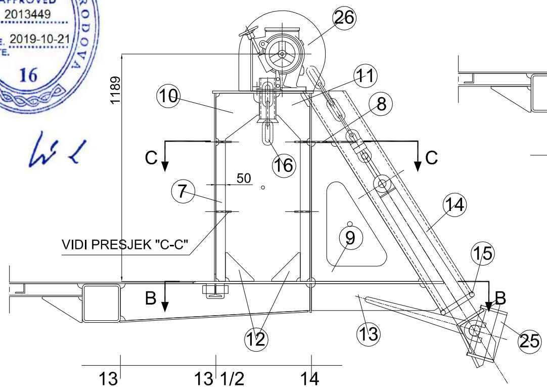
PRIČVRŠĆENJE LANCA ZA LANČANIK, NA LIJEVOM BOKU LANČANIKA
