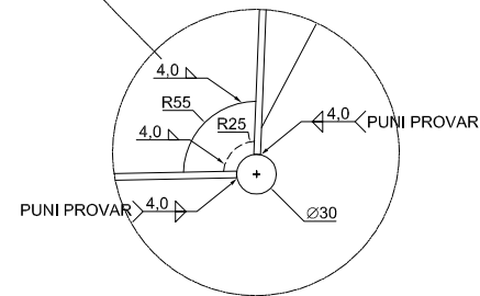
PRESJEK "D-D"
