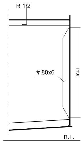
PRESJEK "C-C"
