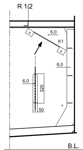
PRESJEK "D-D"
